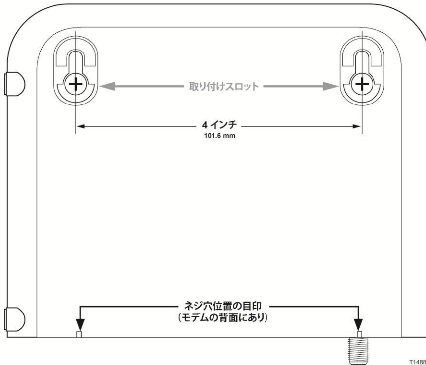
DPC/EPC3008 壁取り付けテンプレート
