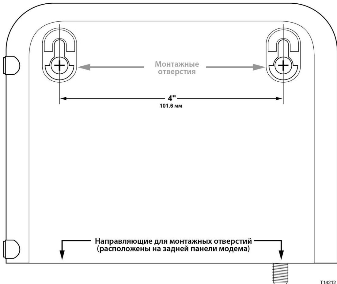
Схема настенного монтажа DPC3010
