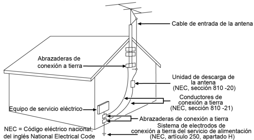
Ejemplo de conexión a tierra de la antena
